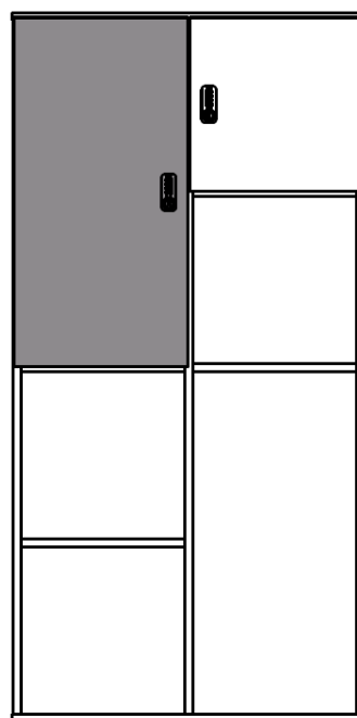
Casier double : H: 780mm L: 377mm P: 377mm
